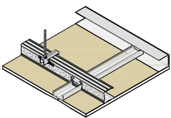
PERFIL PRIMARIO, SECUNDARIO Y PERIMETRAL PLADUR® NEO
